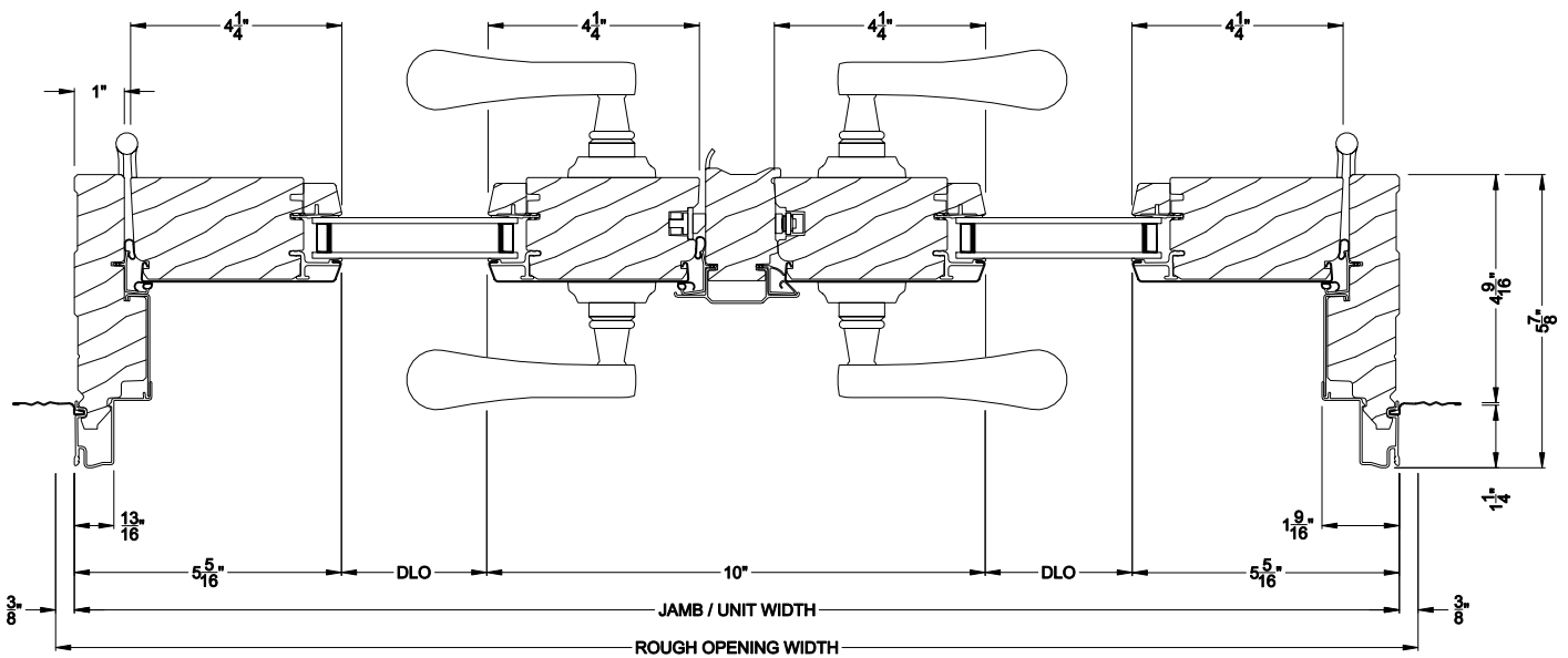
CLASSIC SERIES INSWING DOOR Horizontal Section - Double Door
